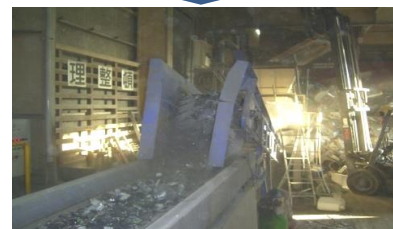
産業廃棄物破碎ライン
