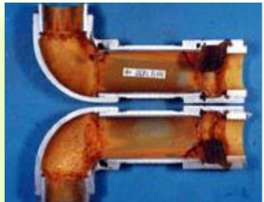
■給水管の抜管調査
